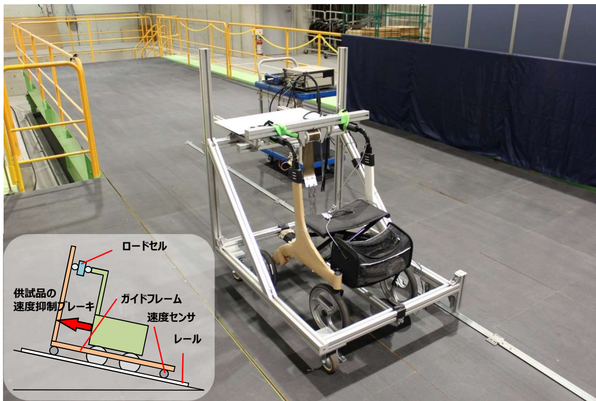
速度抑制機能 試験装置 (供試品のブレーキ能力を計測できます)
