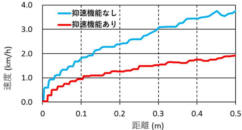
速度抑制機能 計測例 (この計測結果は表頁の製品とは異なります)
