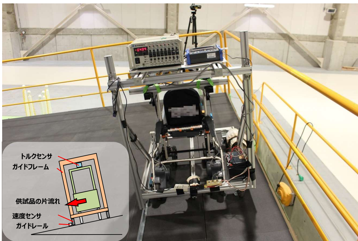
片流れ抑制機能 試験装置 (供試品の片流れの力を計測できます)
